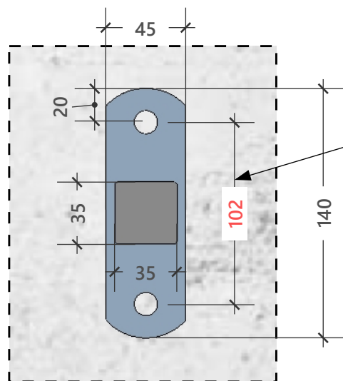
Dettaglio piastra piantone Vista dall'alto
